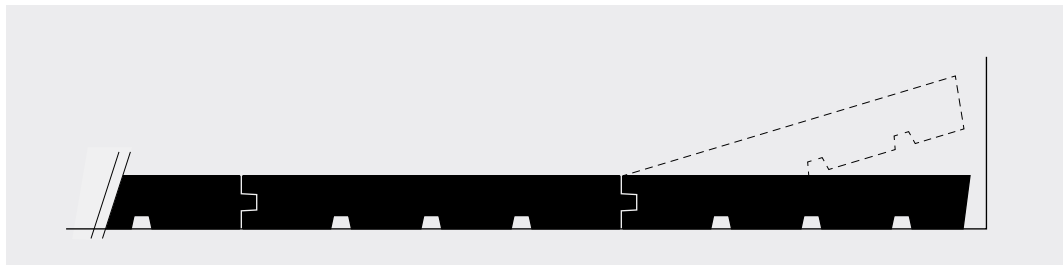
Abbildung 10: Schräger Zuschnitt der letzten Diele zur Wand hin
