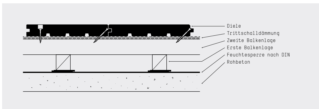
Abbildung 2: Verschraubung auf Balkenlage
