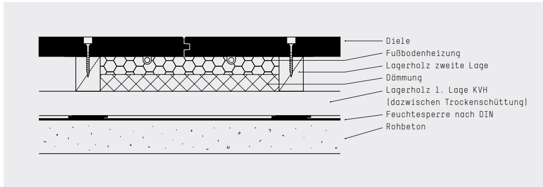
Abbildung 5: Verschraubung auf Trockenbau-Fußbodenheizsystem
