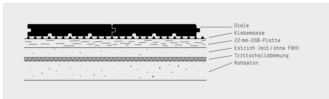
Abbildung 4: Verklebung auf OSB-Platten
