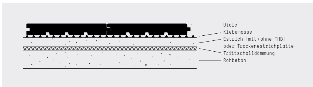
Abbildung 1: Vollflächige Verklebung auf Estrich bzw. Trockenestrich
