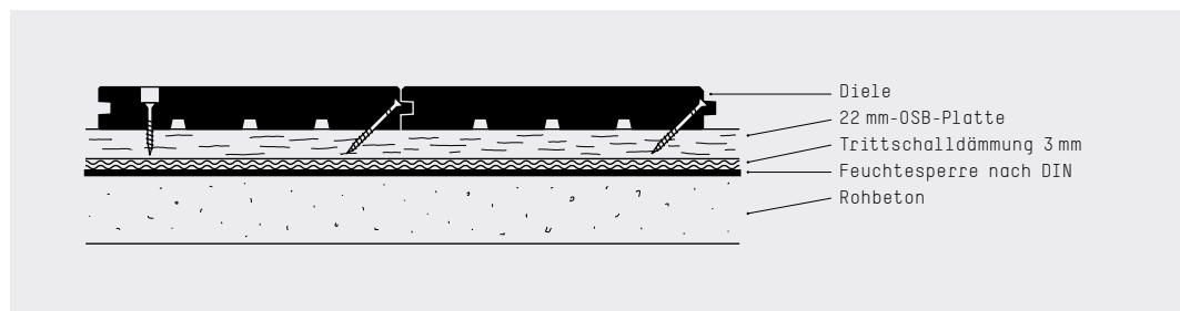
Abbildung 3: Verschraubung auf OSB-Platten
