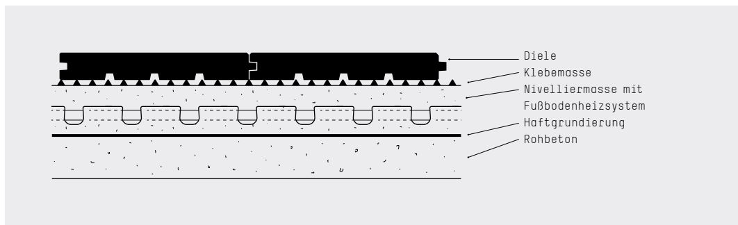
Abbildung 6: Verschraubung auf Dünnschichtestrich-Fußbodenheizsystem
