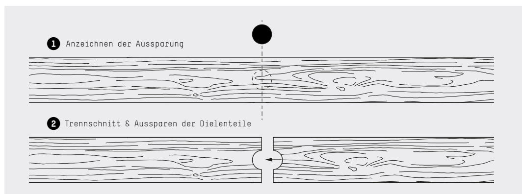
Abbildung 11: Aussparen von Dielen
