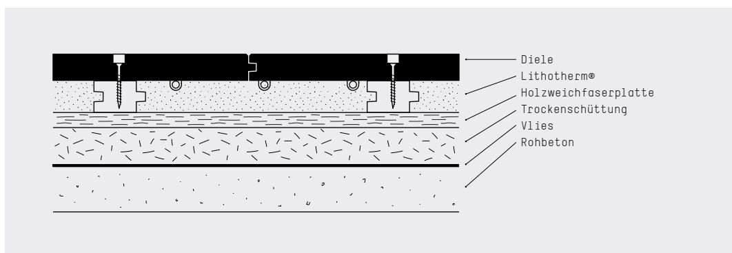
Abbildung 7: Verschraubung auf Lithotherm®
